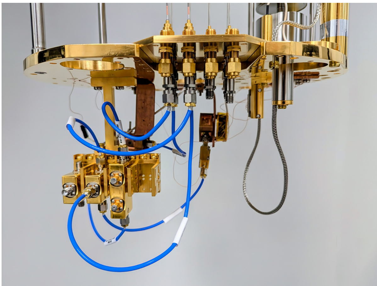
Figura 1: Lo stadio più freddo di un refrigeratore a diluizione recentemente installato presso la Fondazione Bruno Kessler, che raggiunge una temperatura inferiore a 10 millikelvin, su cui sono fissati componenti di elettronica a microonde.
